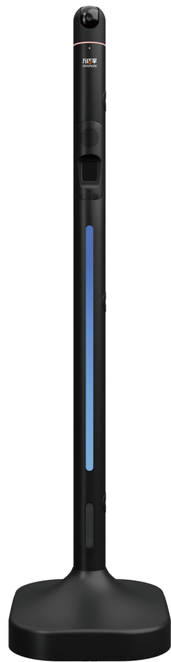
AI机器人
